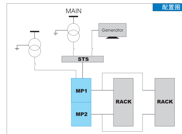
单机柜内双总线方案
