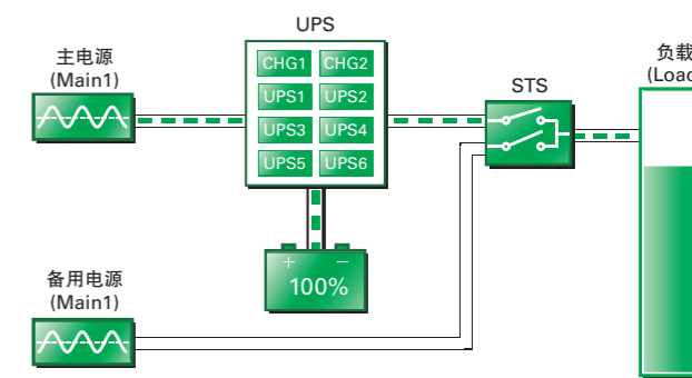
MP 供电示意图
